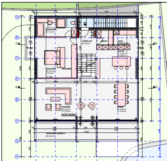
GRUNDRISS OBERGESCHOSS
