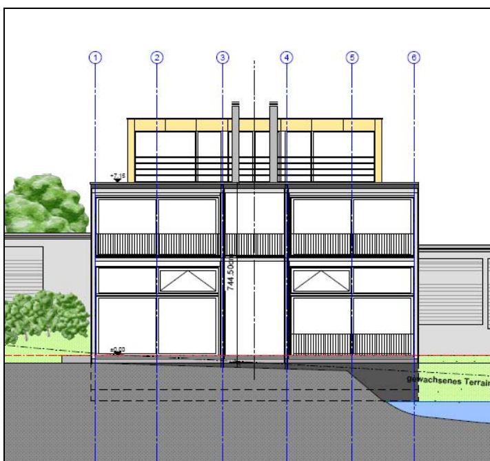
SÜDFASSADE
