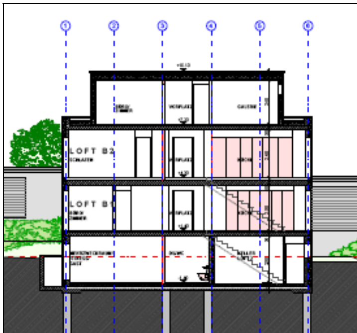
QUERSCHNITT
