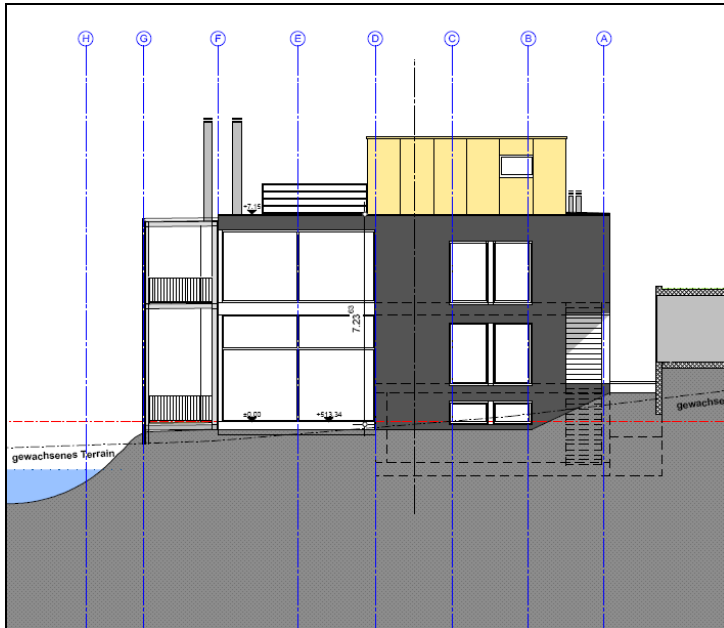
OSTFASSADE
