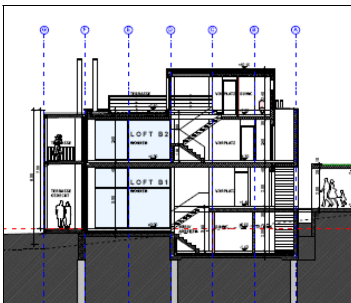
LÄNGSSCHNITT
