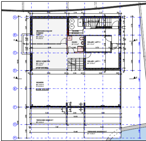
GRUNDRISS UNTERGESCHOSS
