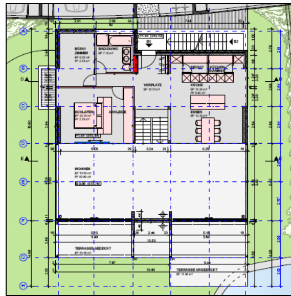
GRUNDRISS ERDGESCHOSS
